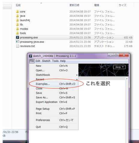
図 5 実行画面
