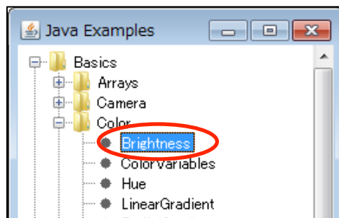
図 6 Brightness の選
