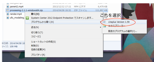
図 4 解凍
